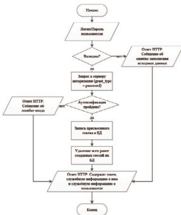
Рис. 3. Блок-схема алгоритма аутентификации пользователя по токenu.
