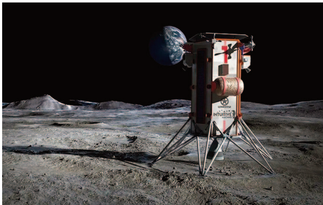
Рис. 5. Лунный ЦОД.
