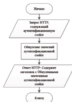
Рис. 2. Блок-схема алгоритма выхода из системы пользователя, авторизованного по cookie.
