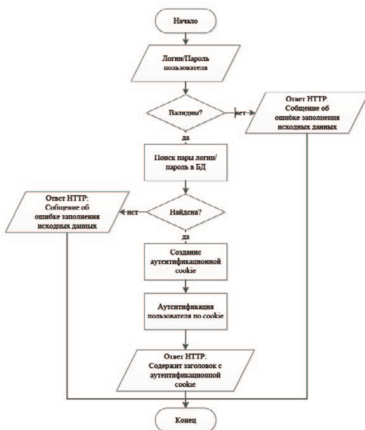
Рис. 1. Блок-схема алгоритма аутентификации пользователя по cookie.
