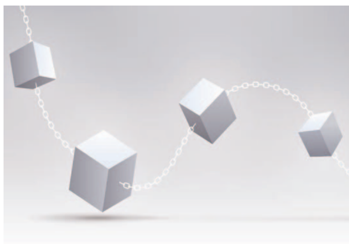
Рис. 5. Блокчейн.
